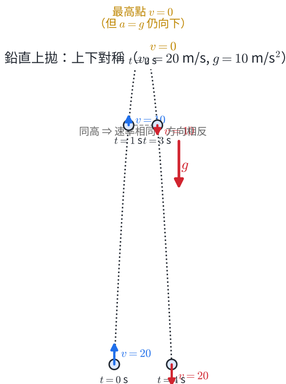
圖 2-2：鉛直上拋的對稱性 ( v_0 = 20 \text{ m/s} , g = 10 \text{ m/s}^2 )。最高點 v = 0 ，但 a = -g 仍向下；同一高度在 t = 1 \text{ s} (上升) 與 t = 3 \text{ s} (下降) 各被經過一次，速率相同、方向相反； t = 0 \text{ s} 拋出 ( v = 20 向上) 與 t = 4 \text{ s} 回到拋出點 ( v = 20 向下) 速率相同。
