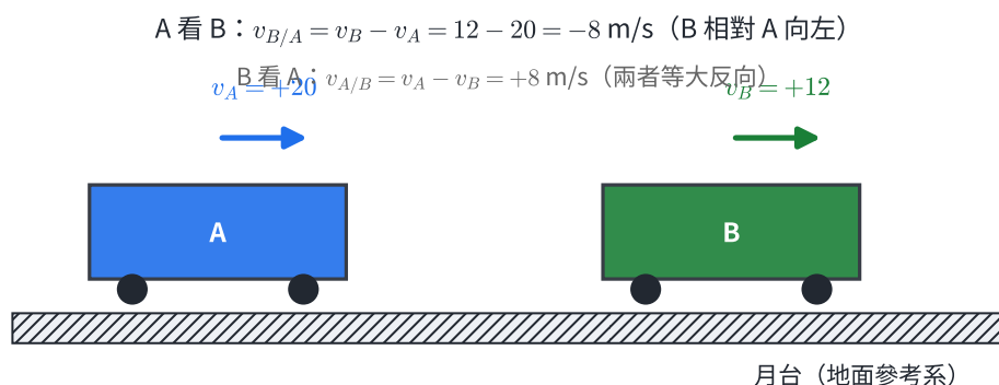
圖 2-3：一維相對速度。A 車 +20 \text{ m/s} 、B 車 +12 \text{ m/s} 同向行駛（向右為正）。A 上的人看 B： v_{B/A} = 12 - 20 = -8 \text{ m/s} （B 相對 A 向左退）；B 上的人看 A： v_{A/B} = 20 - 12 = +8 \text{ m/s} 。兩者等大反向。
